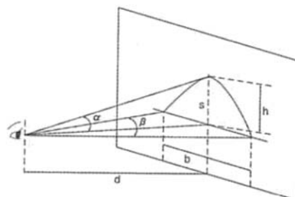
図8 見込角の概念
